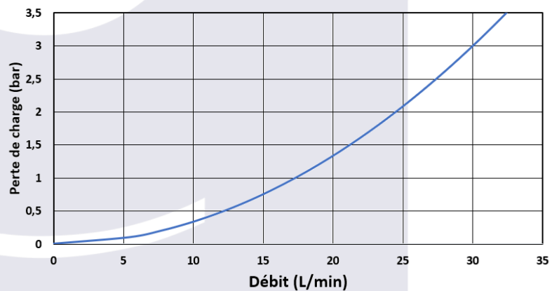
COURBE DE DEBIT
