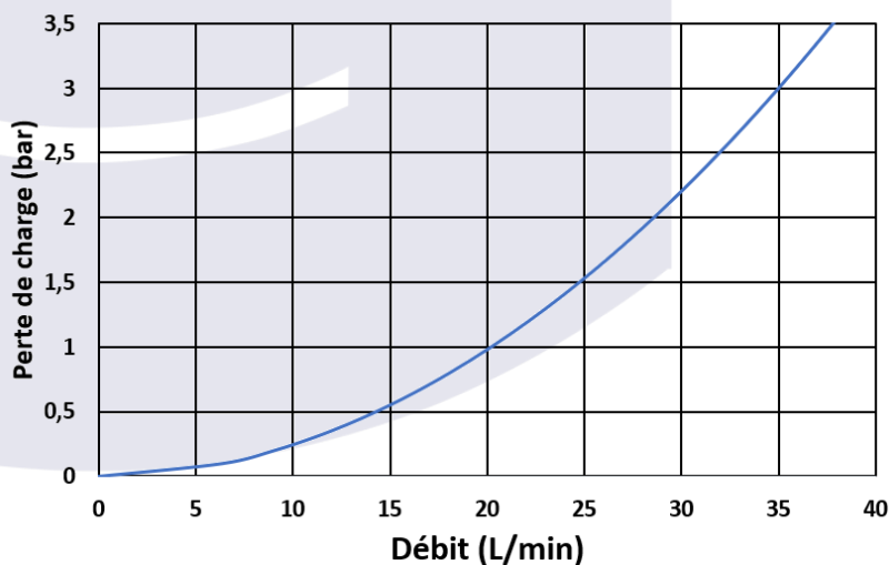
COURBE DE DEBIT
