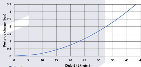
COURBE DE DEBIT
